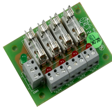
Fused Output Module - 4 Way
